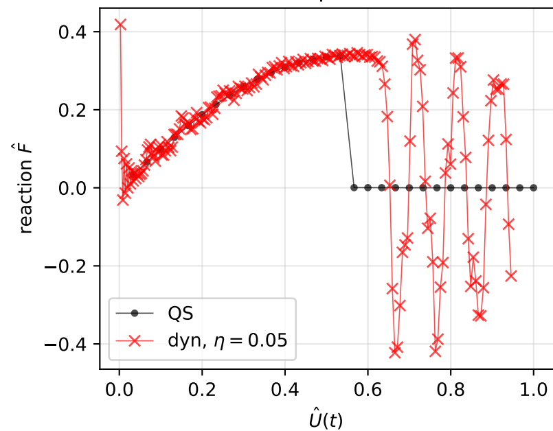
Force-displacement
