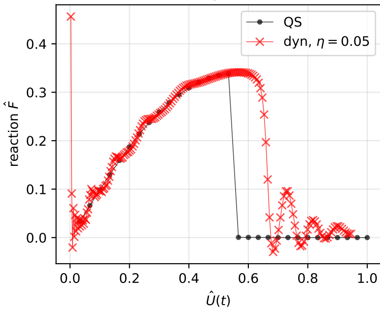
Force-displacement
