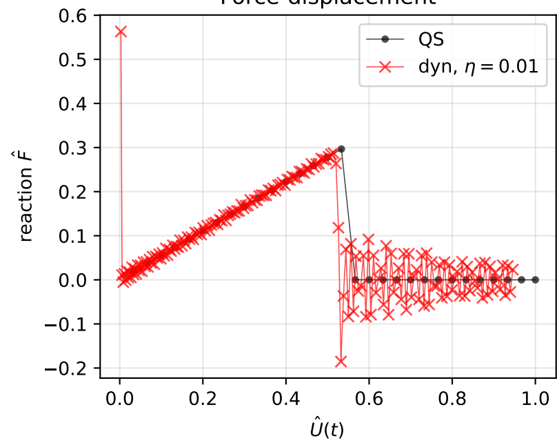
Force-displacement
