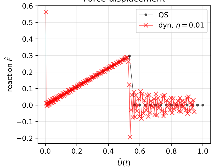
Force-displacement
