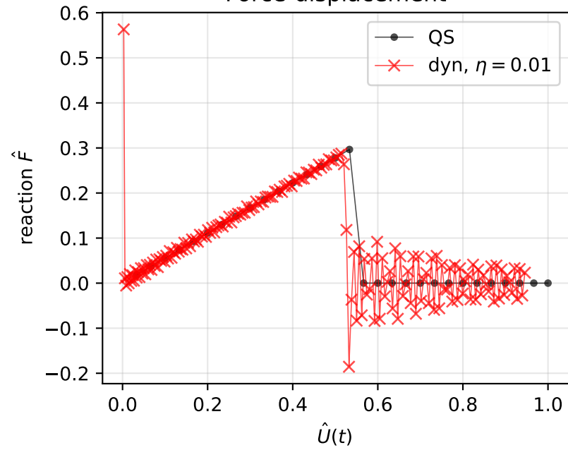
Force-displacement
