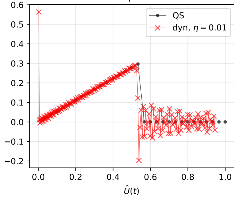
Force-displacement
