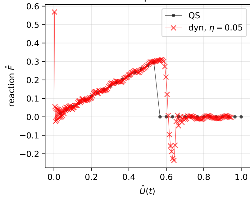
Force-displacement
