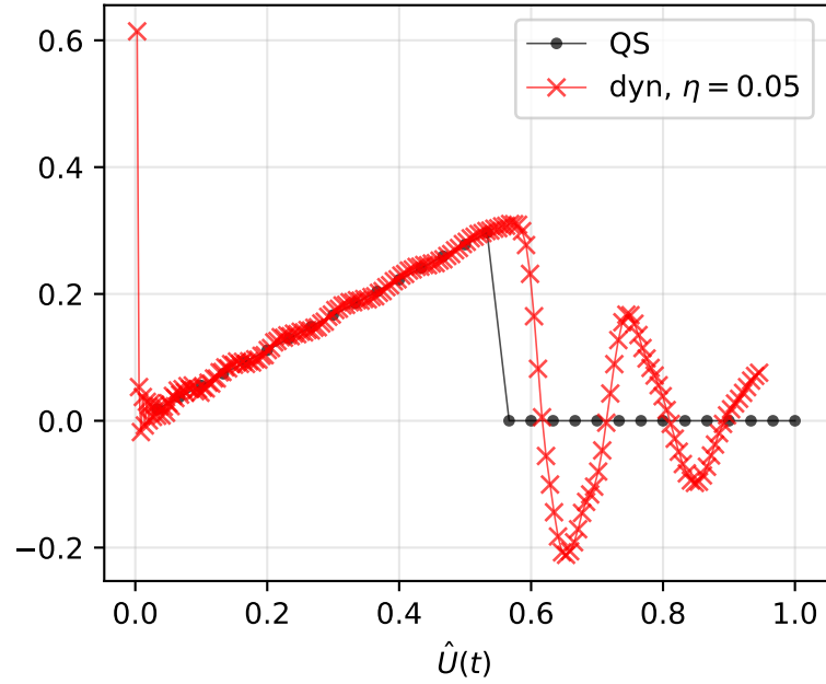
Force-displacement
