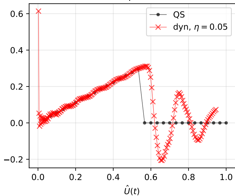
Force-displacement
