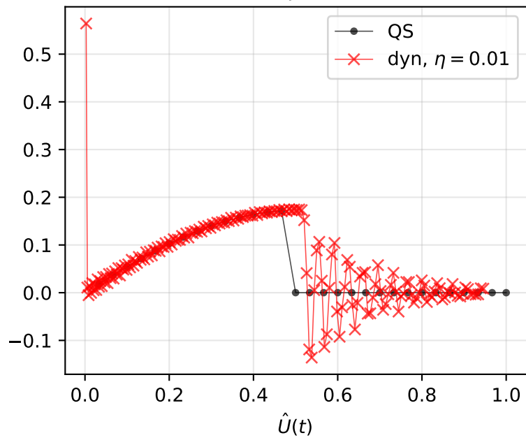
Force-displacement
