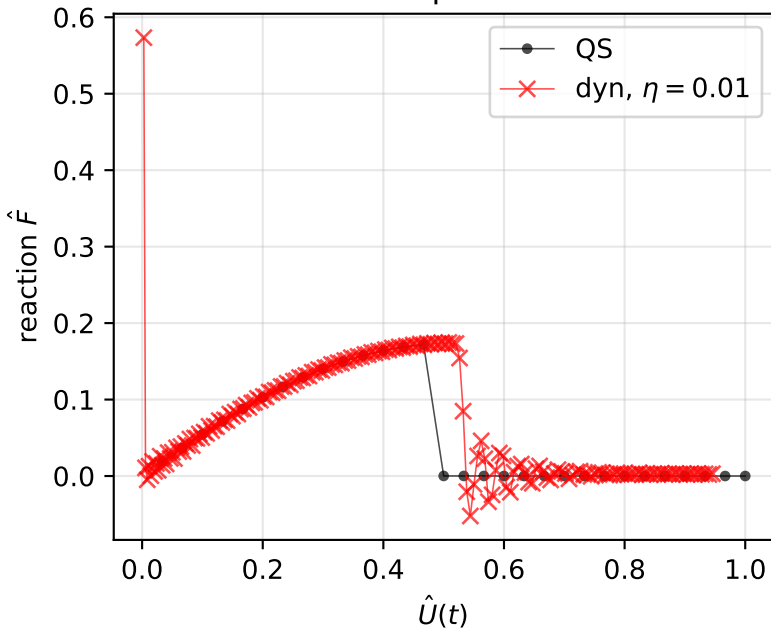
Force-displacement
