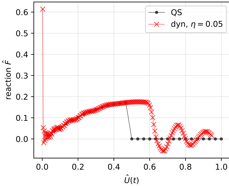
Force-displacement
