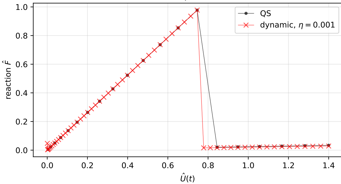
Force-displacement
