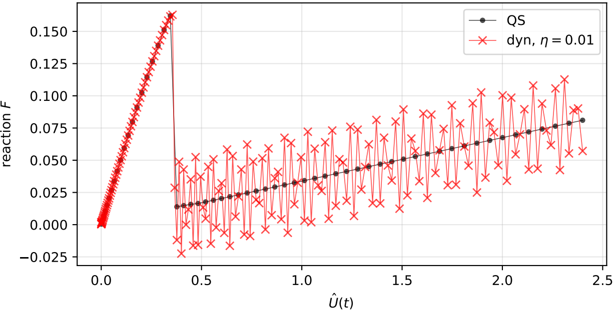
Force-displacement
