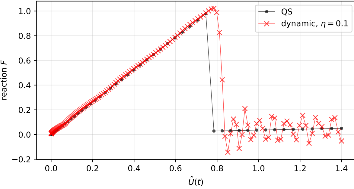
Force-displacement
