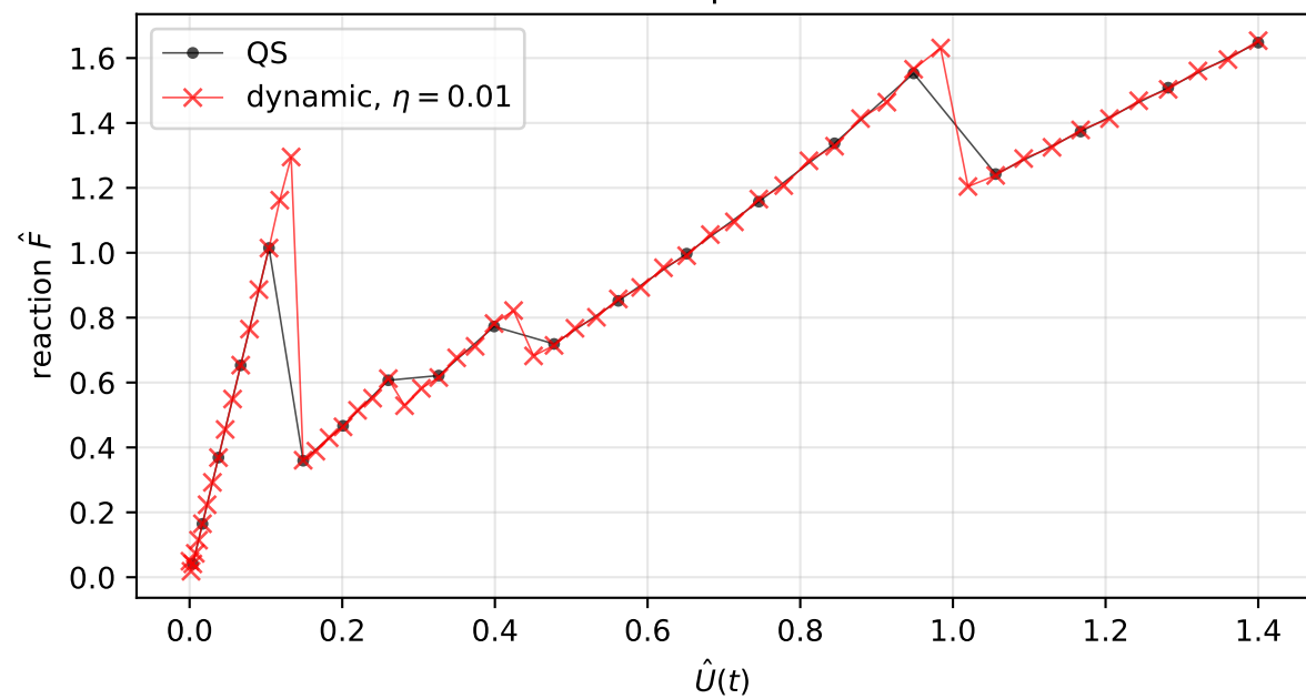
Force-displacement
