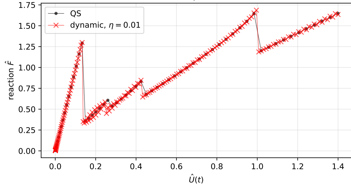
Force-displacement
