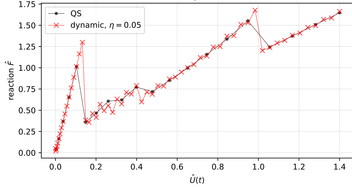
Force-displacement
