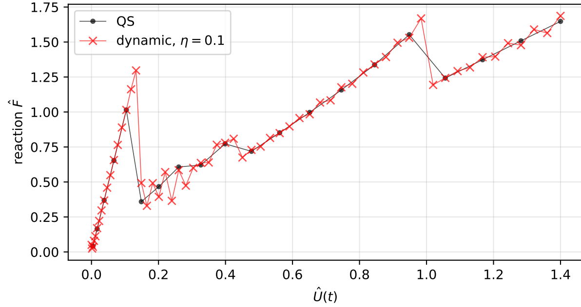
Force-displacement
