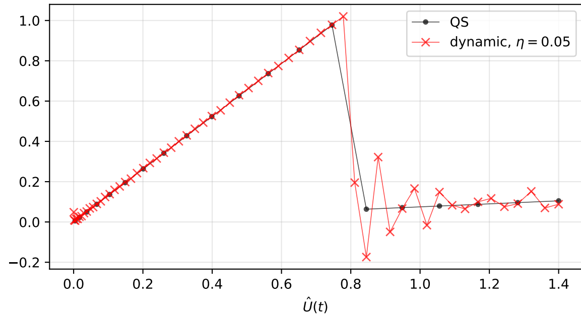
Force-displacement
