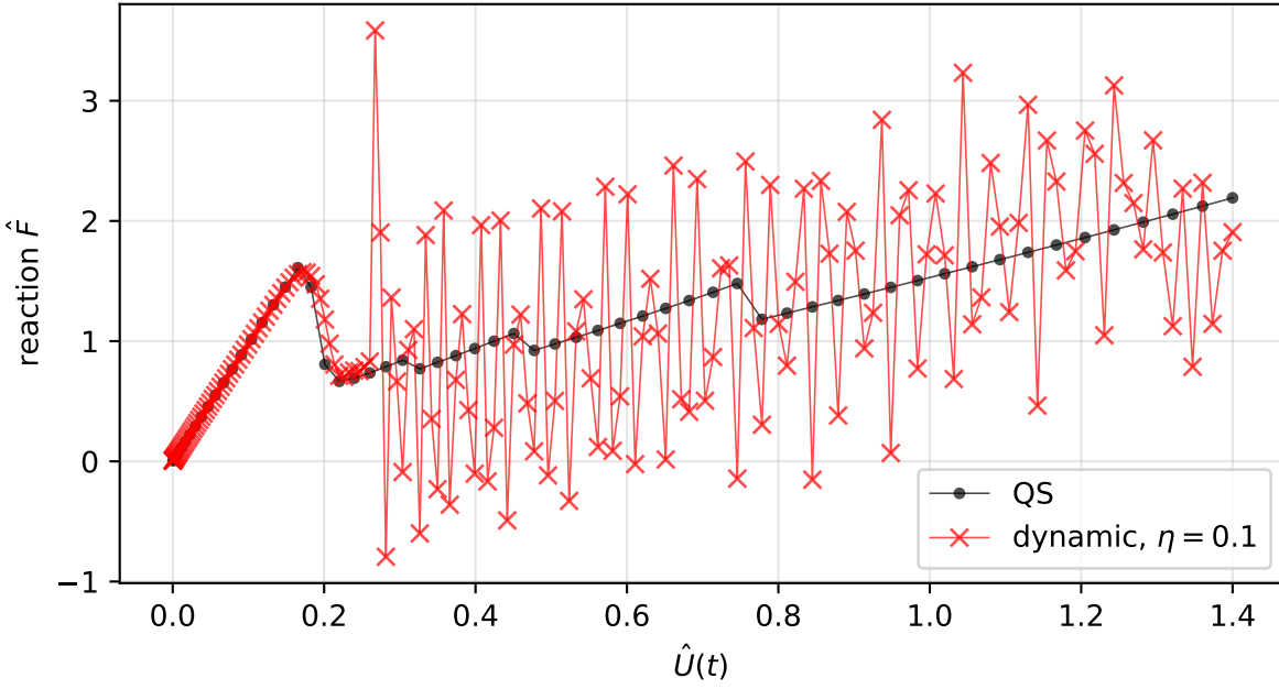
Force-displacement
