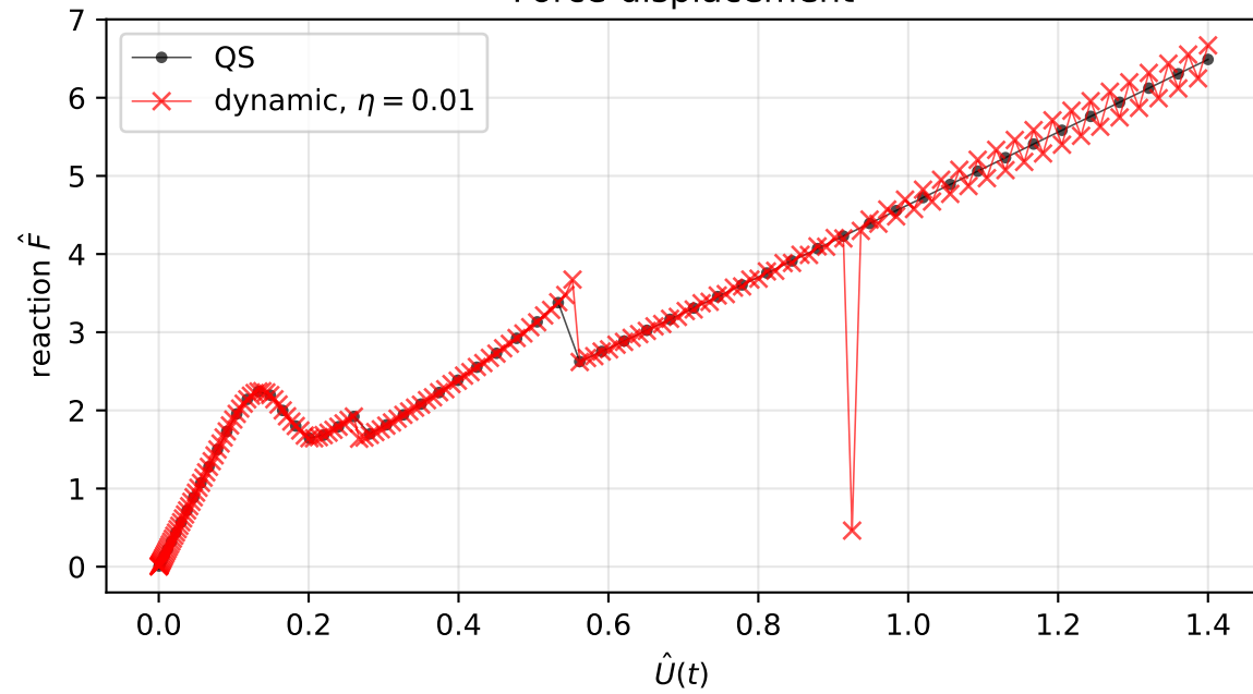
Force-displacement
