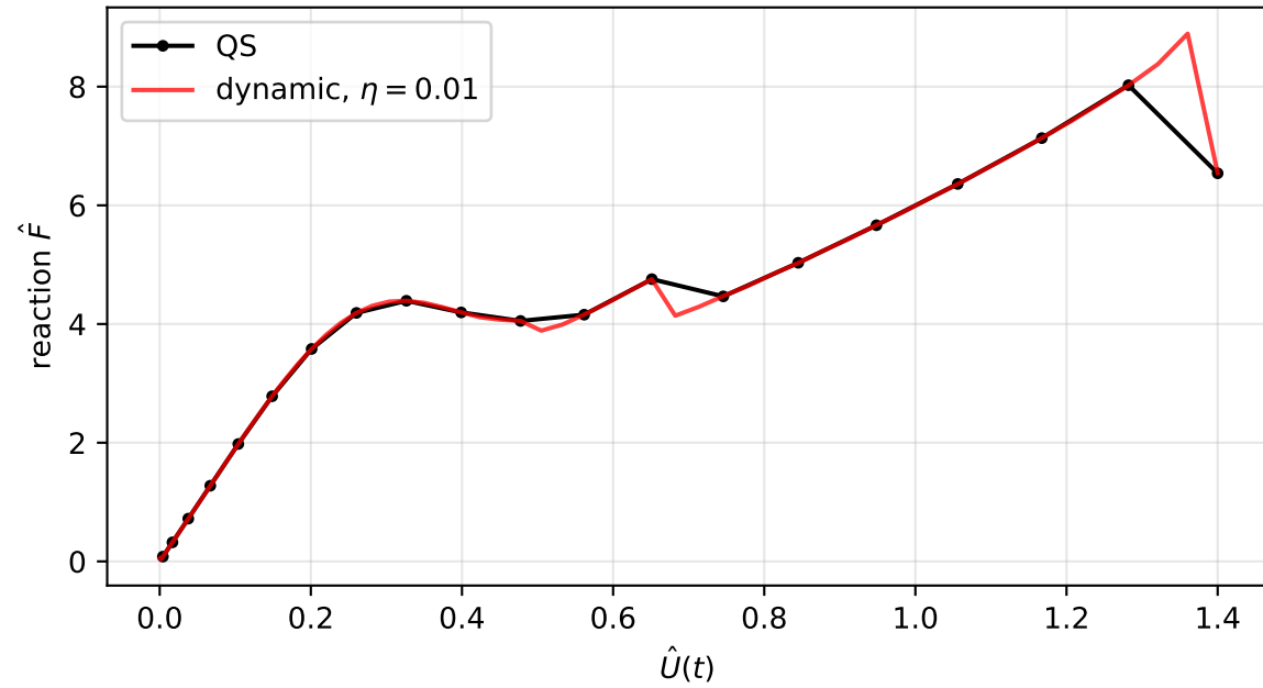
Force-displacement
