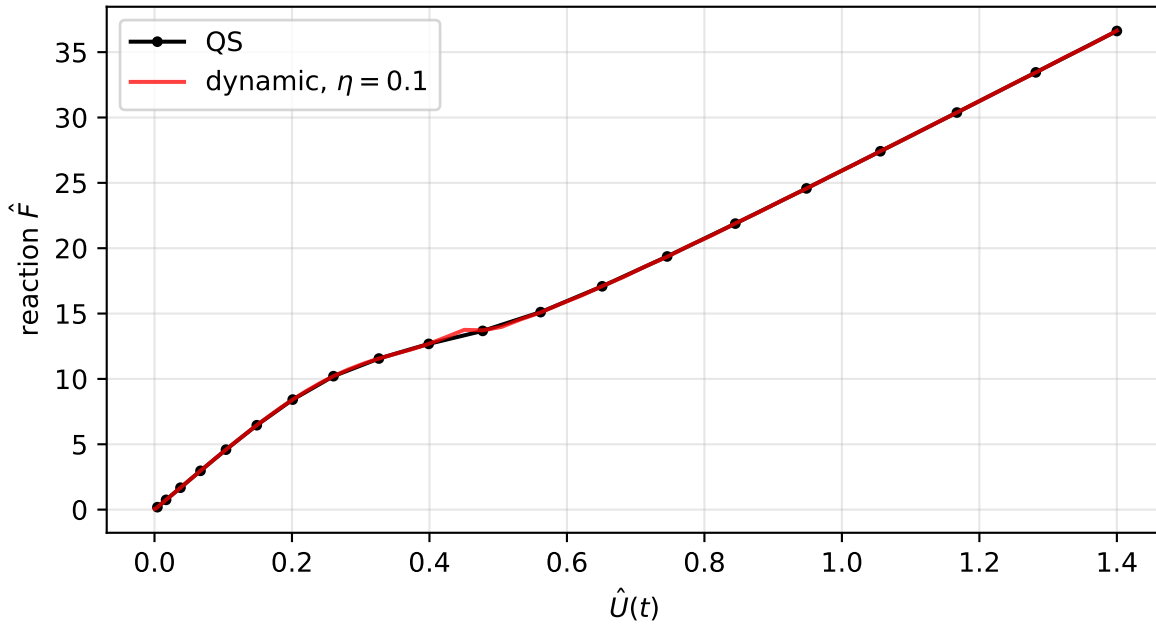
Force-displacement
