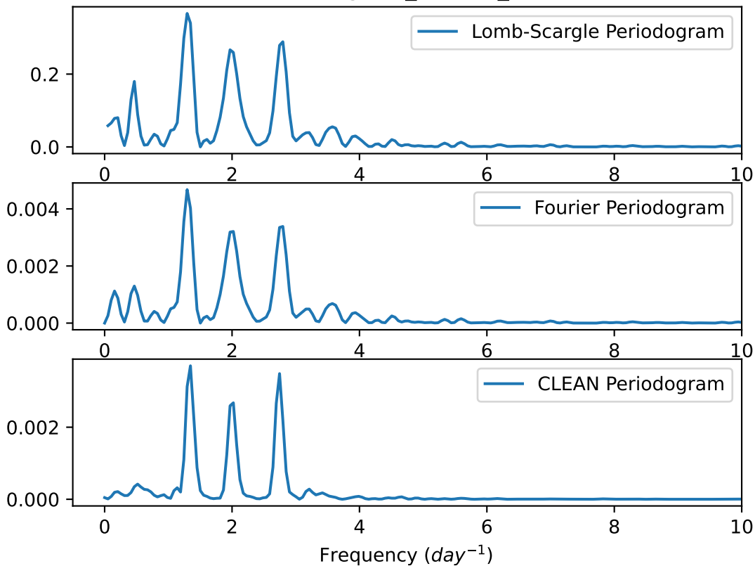
Periodogram_ID1919_001
