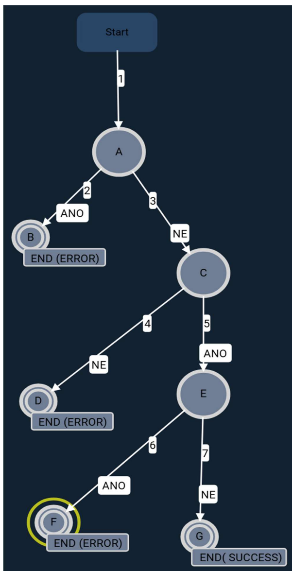
Obrázek 1: Orientovaný graf procesu cancelReservation()
