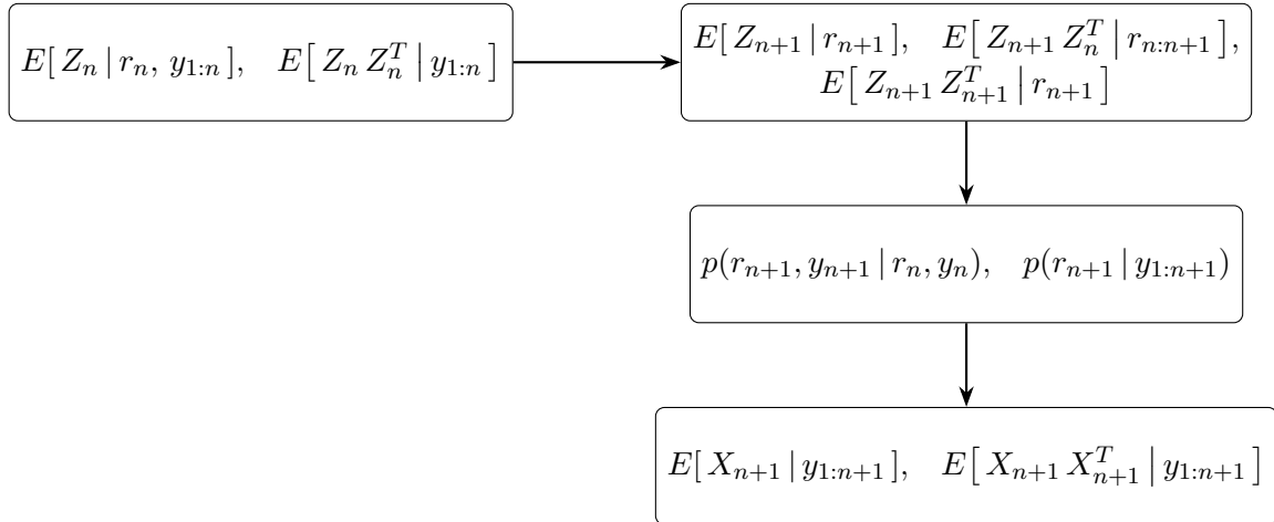
FIGURE 1 – Calcul récursif du filtre optimal et de son erreur quadratique
