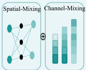
② GaussRWKV
