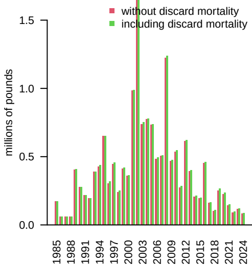
Hire_NNC
