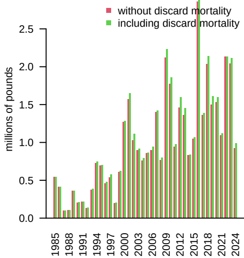
Rec_NNC
