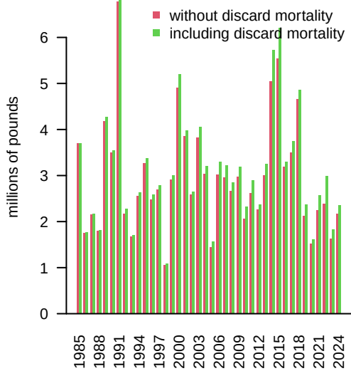
Rec_NCFL
