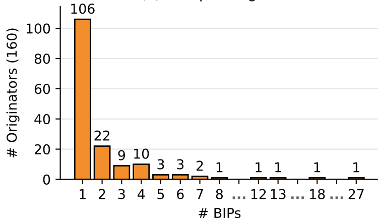
(d) BIPs per Originator
