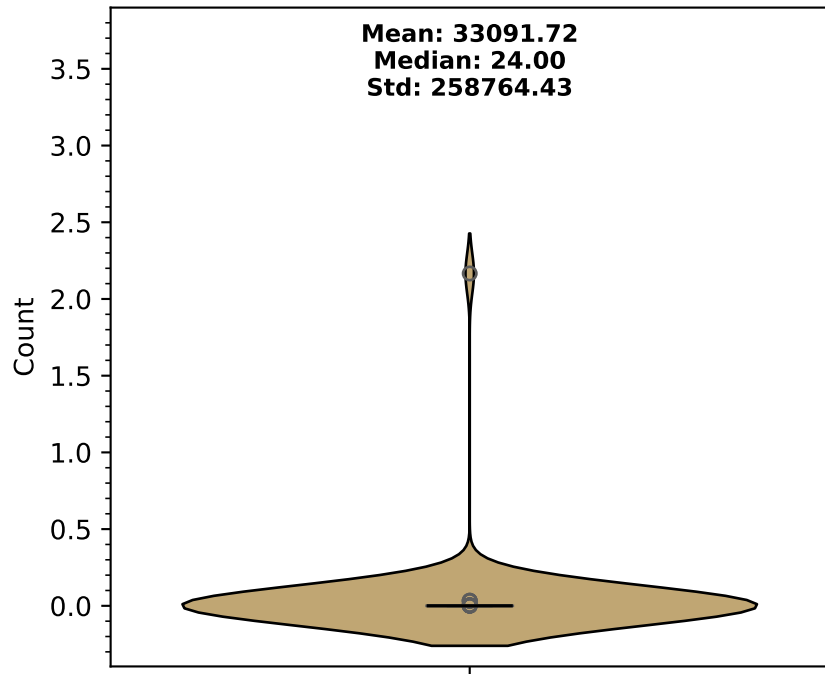
1e6 transition_counts
