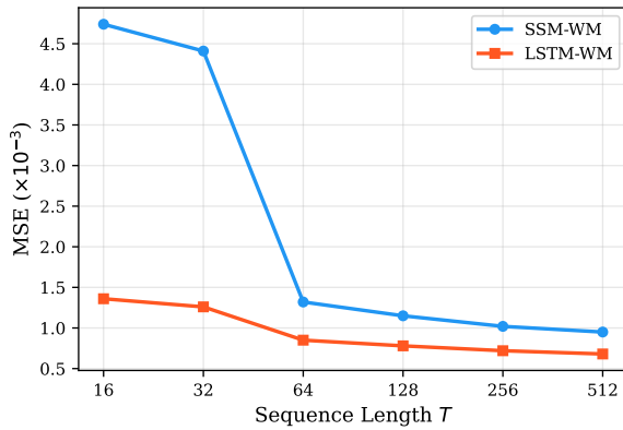
图 4 预测 MSE 随序列长度变化趋势
