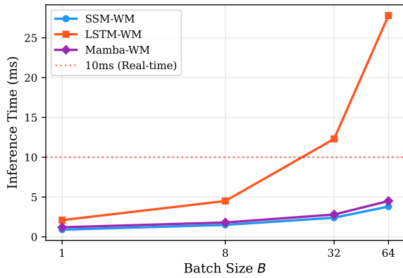
图 2 不同批次大小下的推理时间对比
