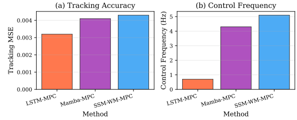
图 7 MPC 控制性能对比
