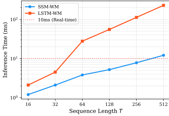
图 3 推理时间随序列长度变化趋势
