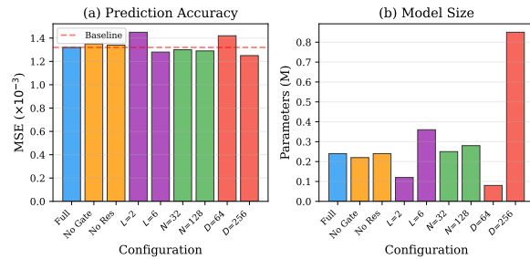
图 5 消融实验结果可视化
