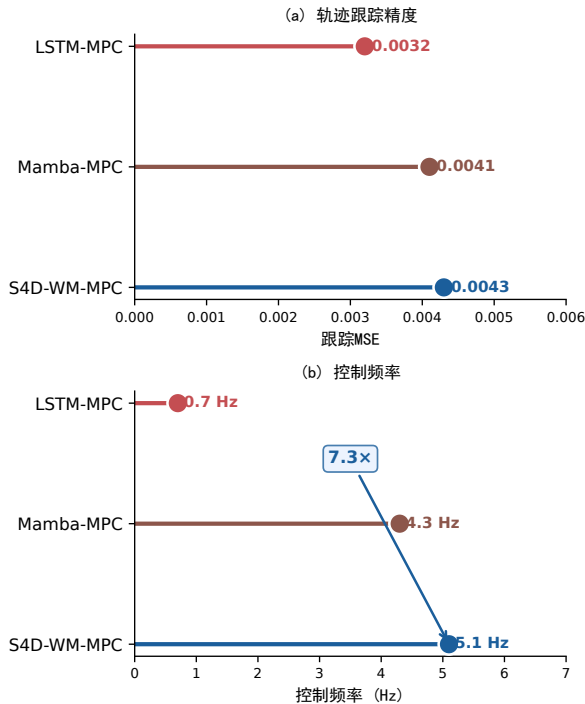
图 5 MPC 控制性能对比
