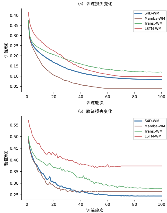
图 4 各模型 D4RL Humanoid 训练曲线
