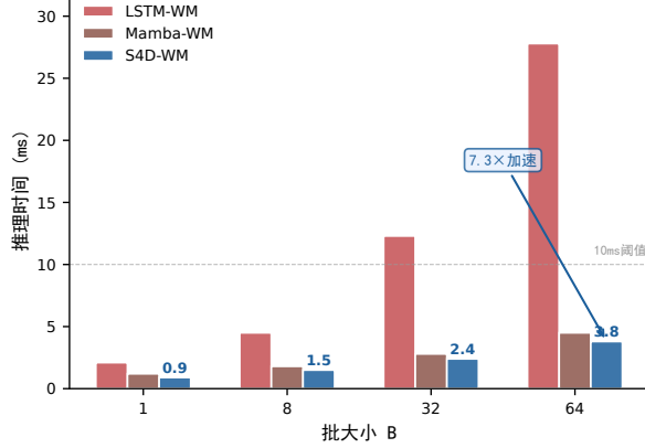
图 1 不同批次大小下的推理时间对比
