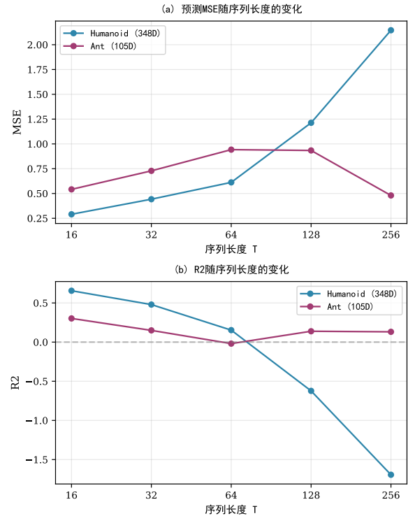
图 2 S4D-WM 在不同序列长度下的预测精度
