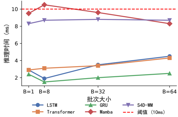
图 2 不同批次大小下的推理时间对比
