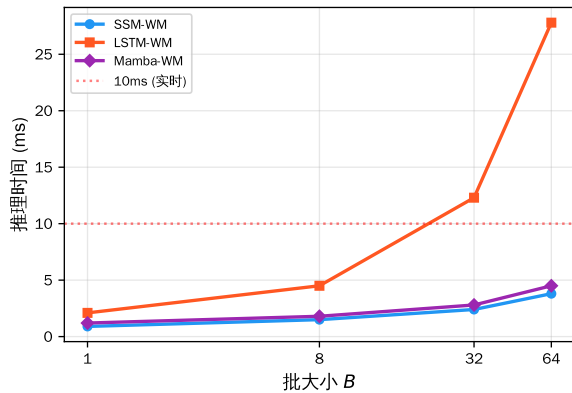
图 1 不同批次大小下的推理时间对比
