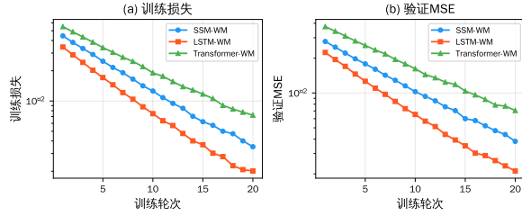
图 5 SSM-WM 训练曲线 (合成数据集)
