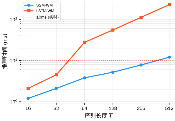
图2 推理时间随序列长度变化趋势
