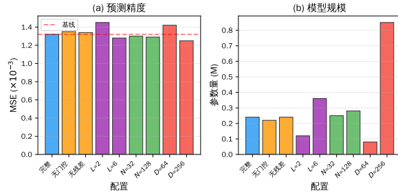
图4 消融实验结果可视化
