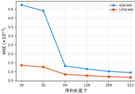
图3 预测 MSE 随序列长度变化趋势
