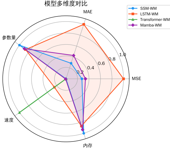
图 7 各方法多维度性能雷达图对比
