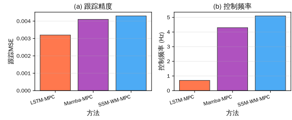
图 6 MPC 控制性能对比
