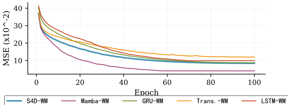
(a) 训练损失
