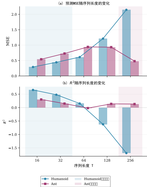
图 3 S4D-WM 在不同序列长度下的预测精度
