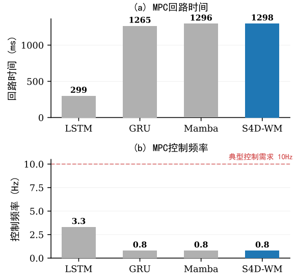
图 7 MPC 控制性能对比
