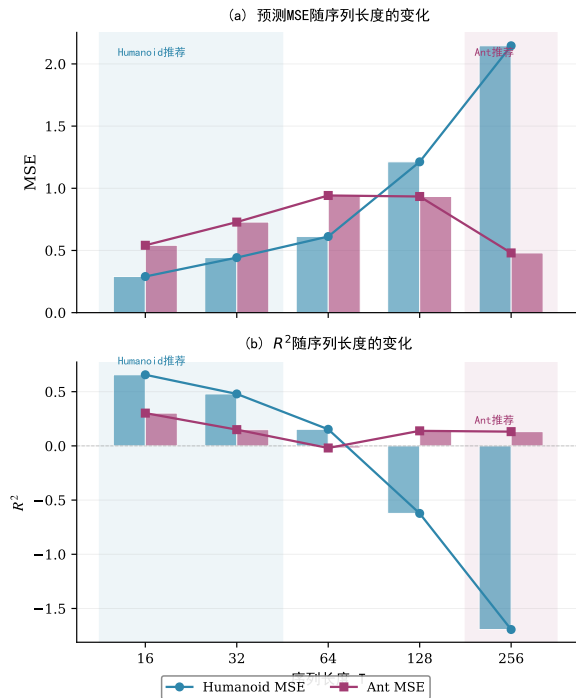
图 3 S4D-WM 在不同序列长度下的预测精度
