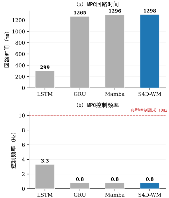
图 6 MPC 控制性能对比
