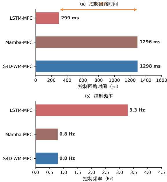
图 5 MPC 控制性能对比
