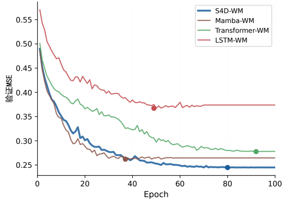
图 4 各模型 D4RL Humanoid 训练曲线
