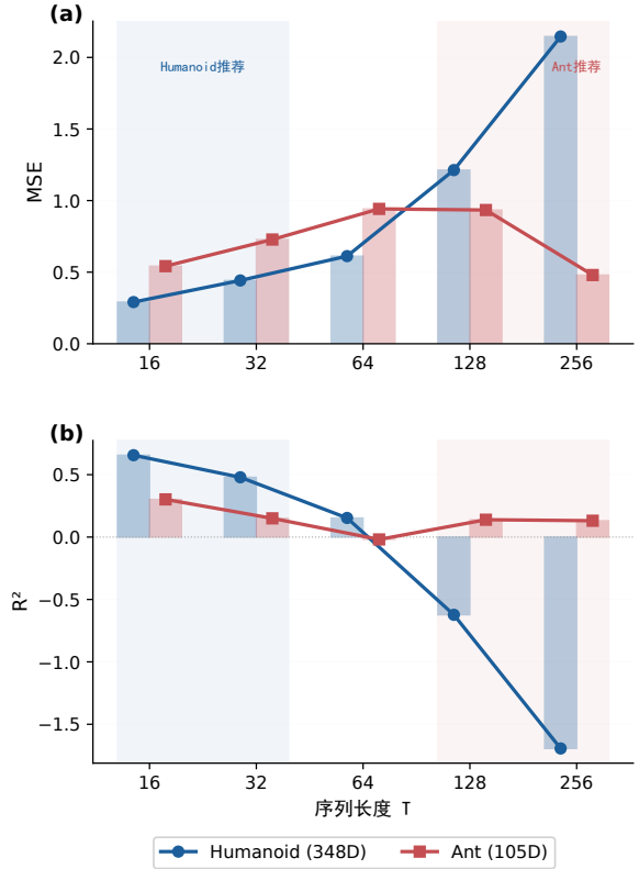
图 2 S4D-WM 在不同序列长度下的预测精度
