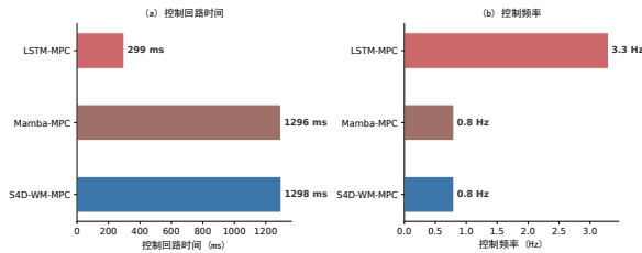
图 5 MPC 控制性能对比
