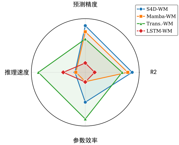
图 6 各方法多维度性能对比 (D4RL Humanoid)
