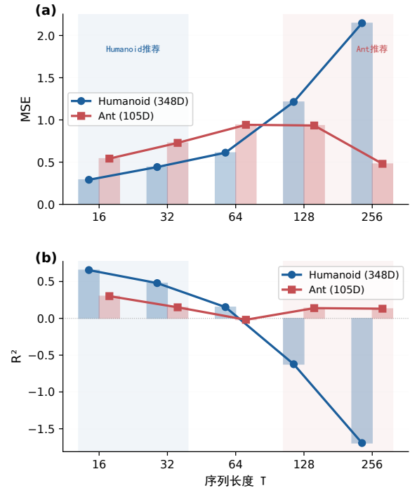
图 2 S4D-WM 在不同序列长度下的预测精度
