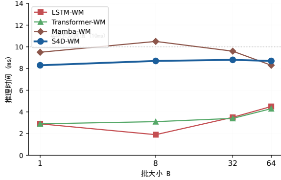
图 1 不同批次大小下的推理时间对比
