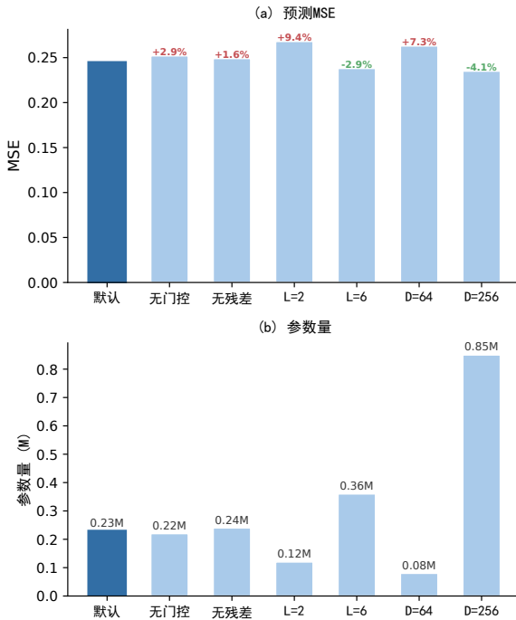
图 3 消融实验结果可视化
