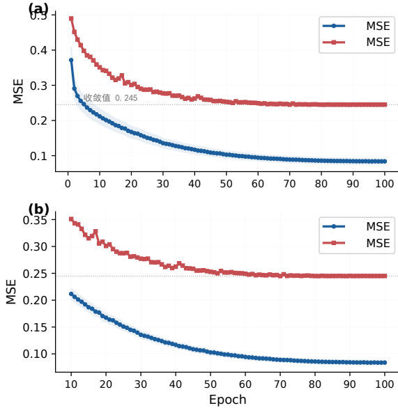
图 4 各模型 D4RL Humanoid 训练曲线
