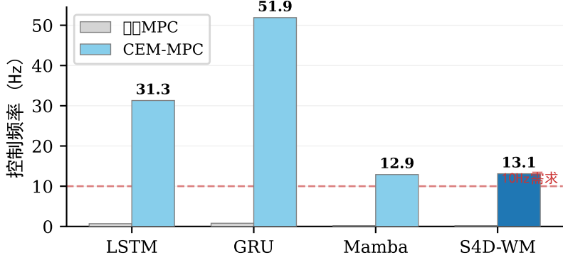
(b) MPC控制频率
