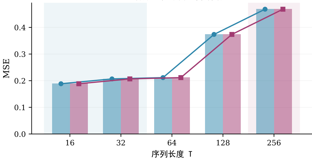
(a) 预测MSE随序列长度的变化
