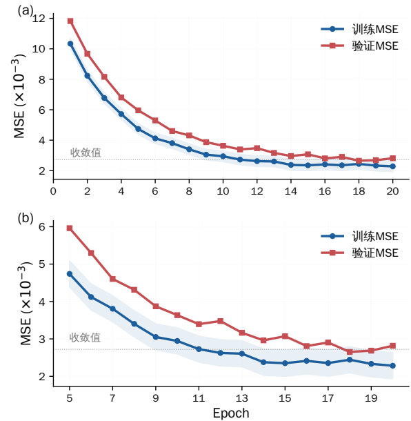
图 4 S4D-WM 训练曲线 (阴影区域表示训练 MSE 的 \pm 标准差)
