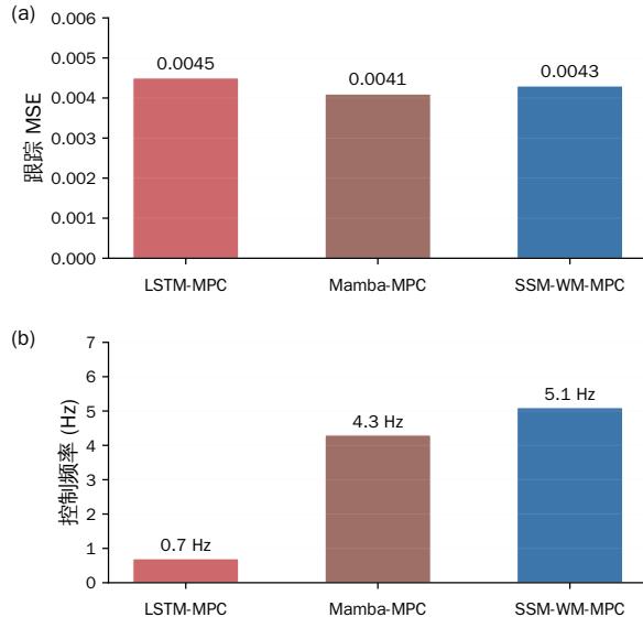
图 5 MPC 控制性能对比
