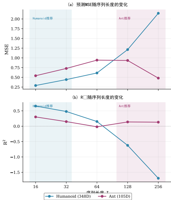
图 3 S4D-WM 在不同序列长度下的预测精度
