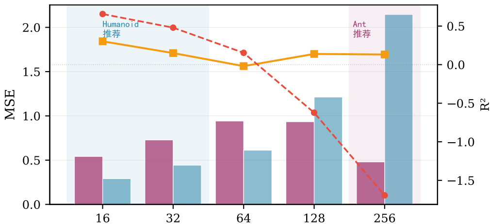
(b) Ant (105维)
