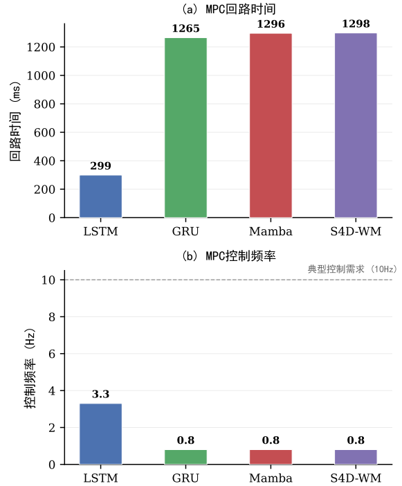
图 6 MPC 控制性能对比
