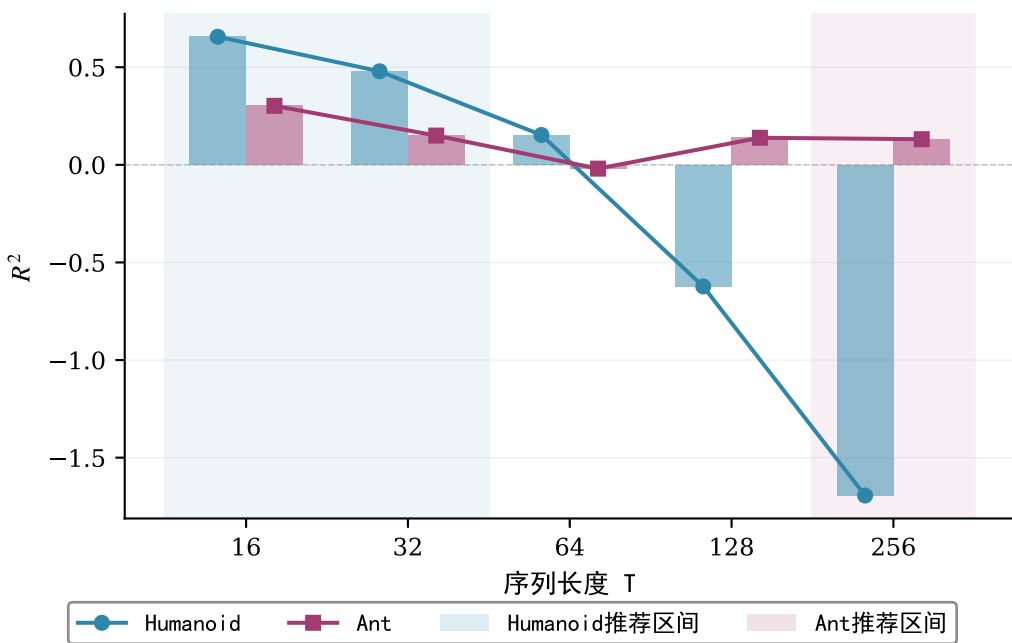
(b) R^2 随序列长度的变化
