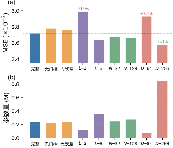
图 3 消融实验结果可视化
